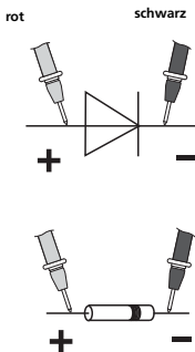
Durchlassrichtung
