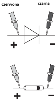
Kierunek przewodzenia
