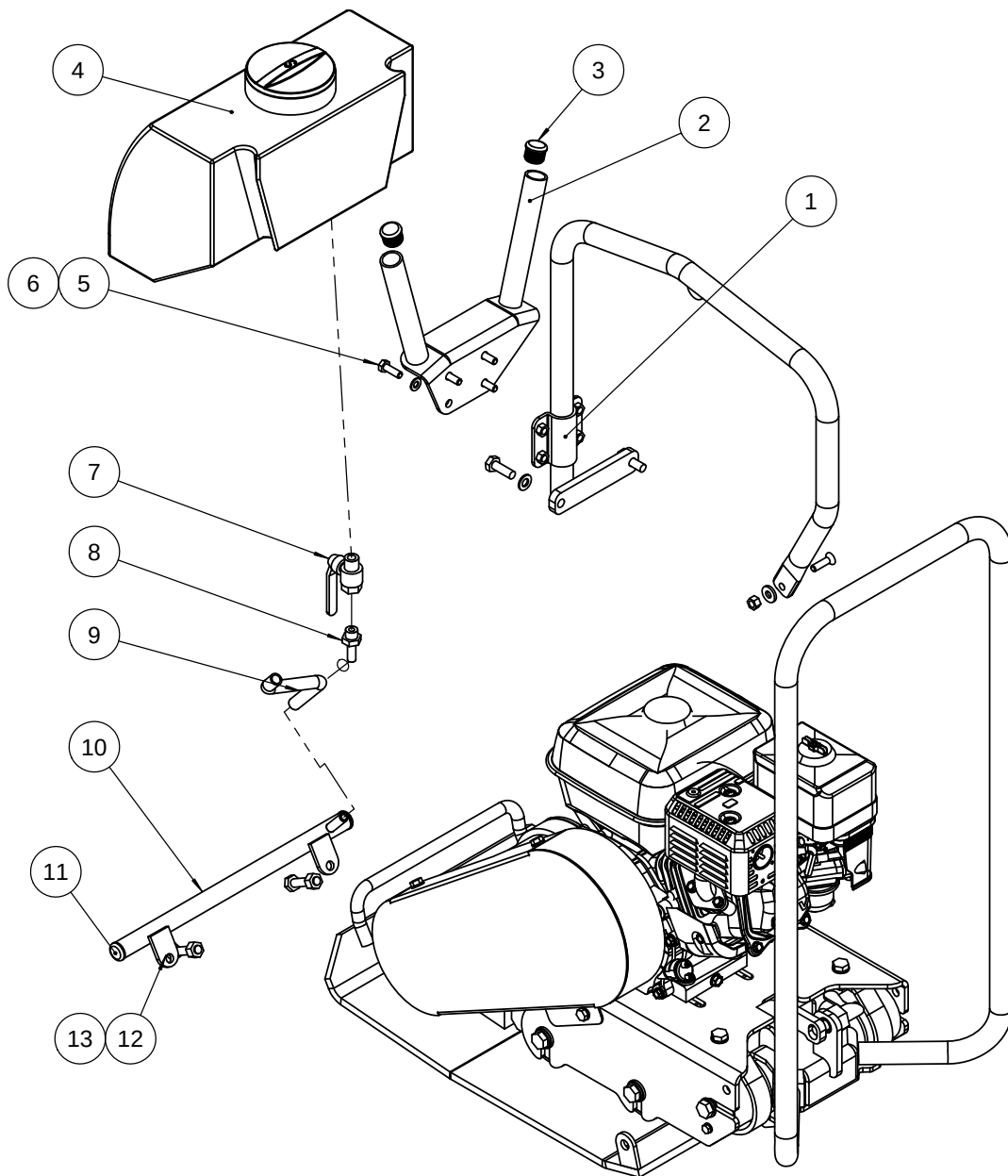
WATER SYSTEM (OPTIONAL) WASSERSYSTEM VANDSYSTEM TANQUE DE AGUA
