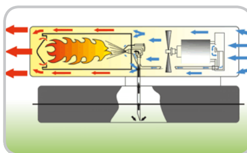
Funktionsprincip
