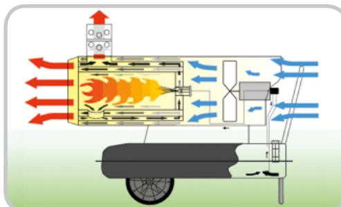
Funktionsprincip
