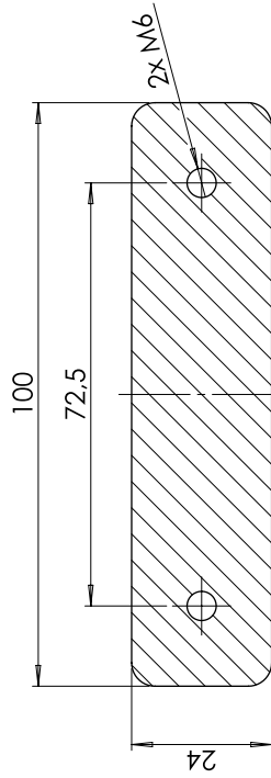
SCHNITT A-A 1 : 1
