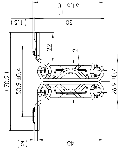
DETAIL Z 1 : 1
